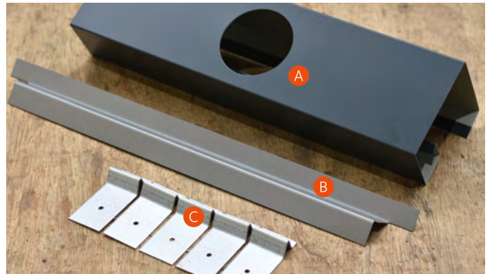
Ein Auszug aus dem Kantteil-Portfolio von ArcelorMittal Construction:
